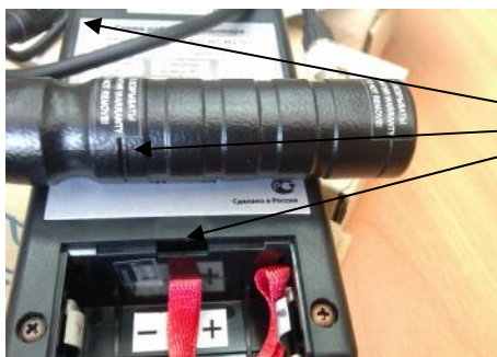
Рисунок 1 – Внешний вид твердомера МЕТ-У1
