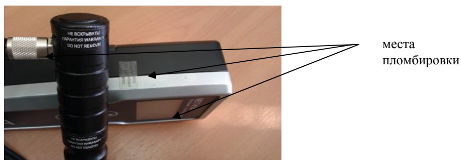
Рисунок 4 - Схема пломбировки твердомера.
